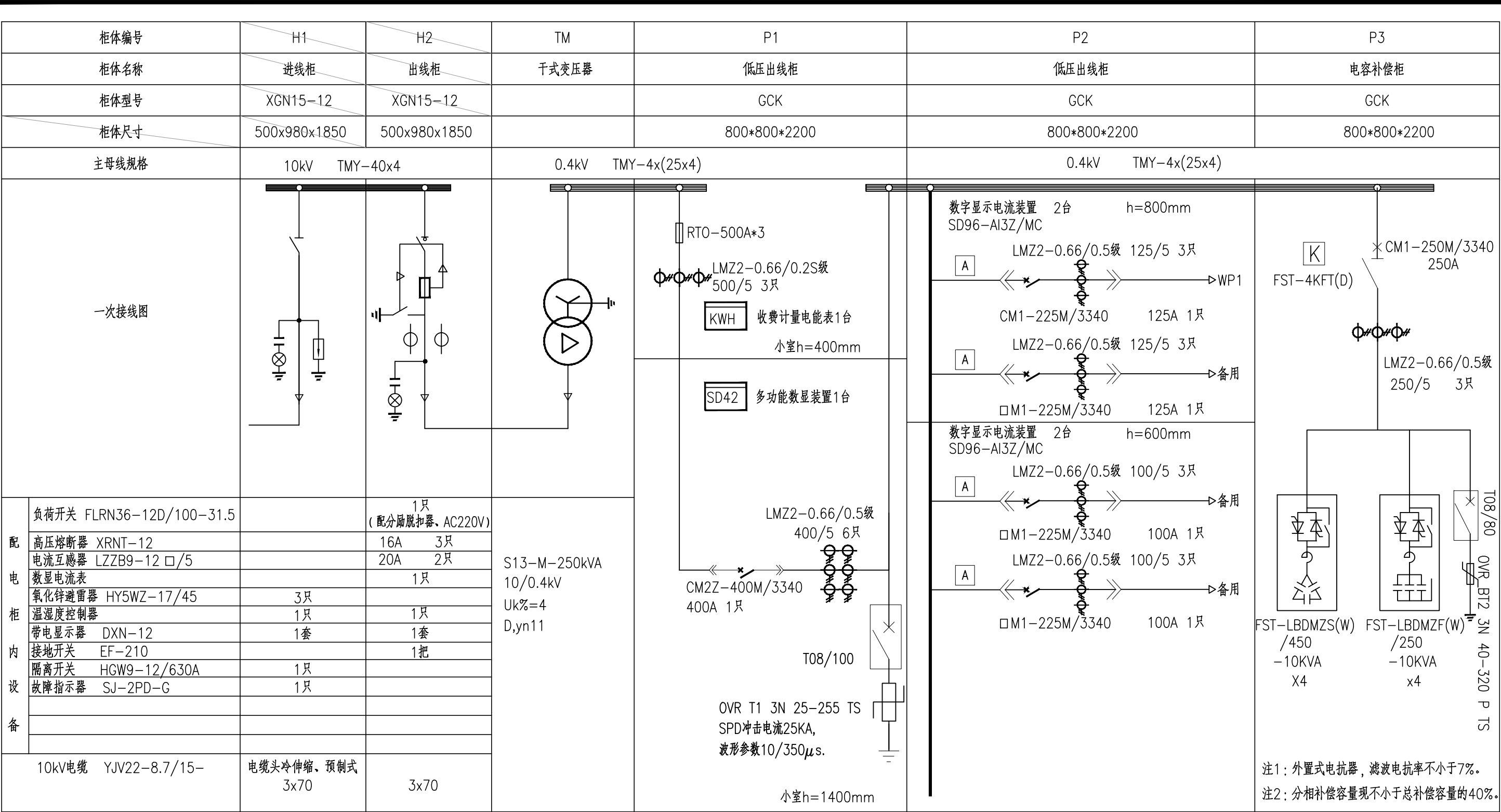
箱变一次变电系统图
